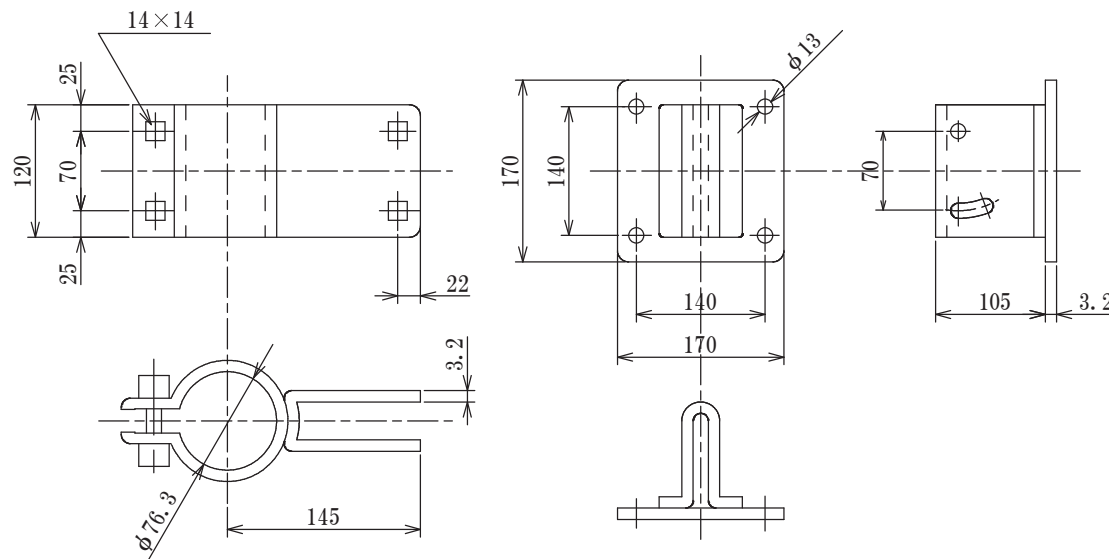
5. 6. 7. 8 取付金具
