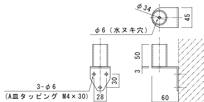
No. 3金具 (壁面用金具) S=1:5
