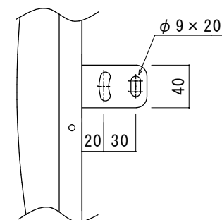
No. 2金具 (支柱用金具: 34φ ~ 50.8φ 対応) S=1:5
