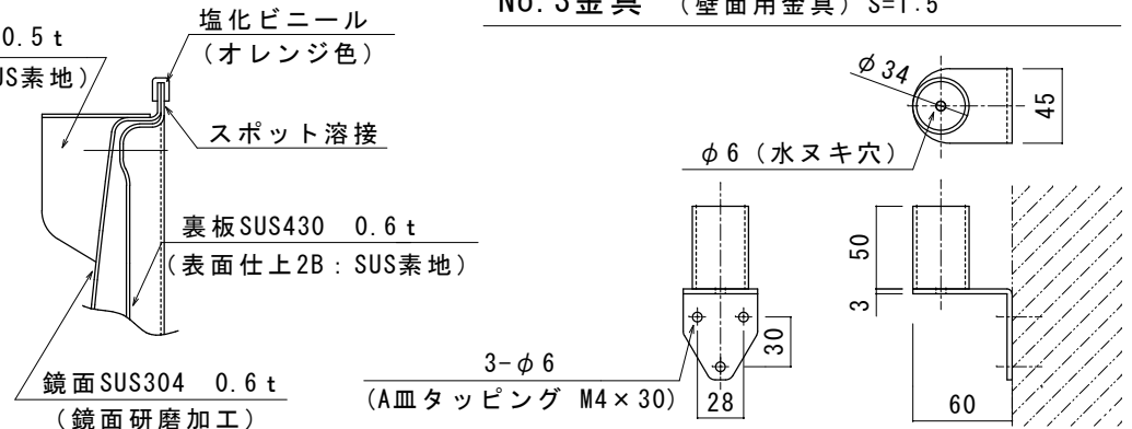
No. 3金具 (壁面用金具) S=1:5
